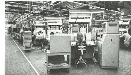
Il reparto delle Gardner Denver per il wire wrap automatico. In primo piano la G.D. « verticale ».
