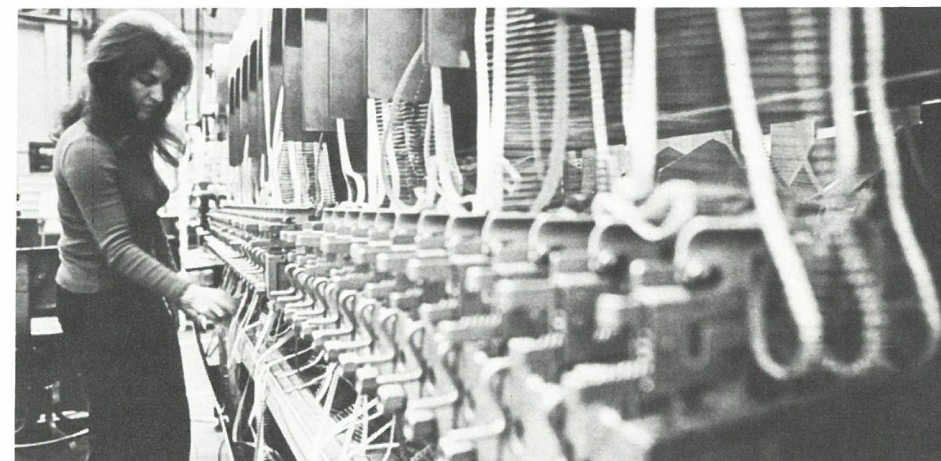
La sequenziatrice automatica di componenti con reofori assiali. La macchina, prelevando componenti da altri nastri sequenzia su di un nuovo nastro i componenti...
